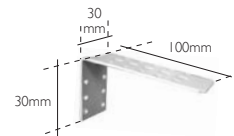
Soporte de instalación a techo
